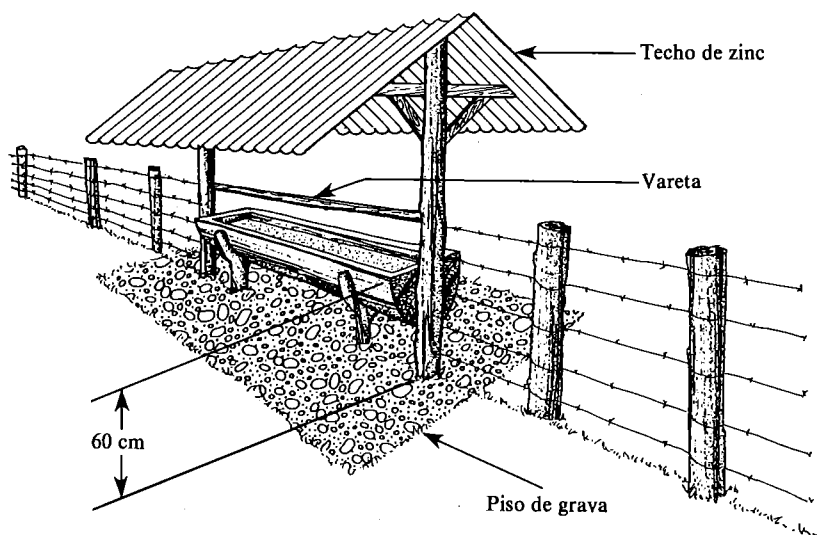
Figura 7. Principales características del saladero. La colocación de éste a lo largo o a través de las cercas permite su utilización simultánea en dos potreros.
