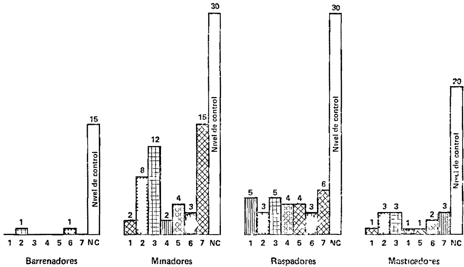
Fig 4 Maximo daño (% hojas o tallos) ocasionado por cuatro diferentes grupos de plagas, durante el ciclo completo de cultivo, determinado en siete campos comerciales del Valle del Cauca en parcelas sin aplicación de insecticidas CIAT 1985 86
