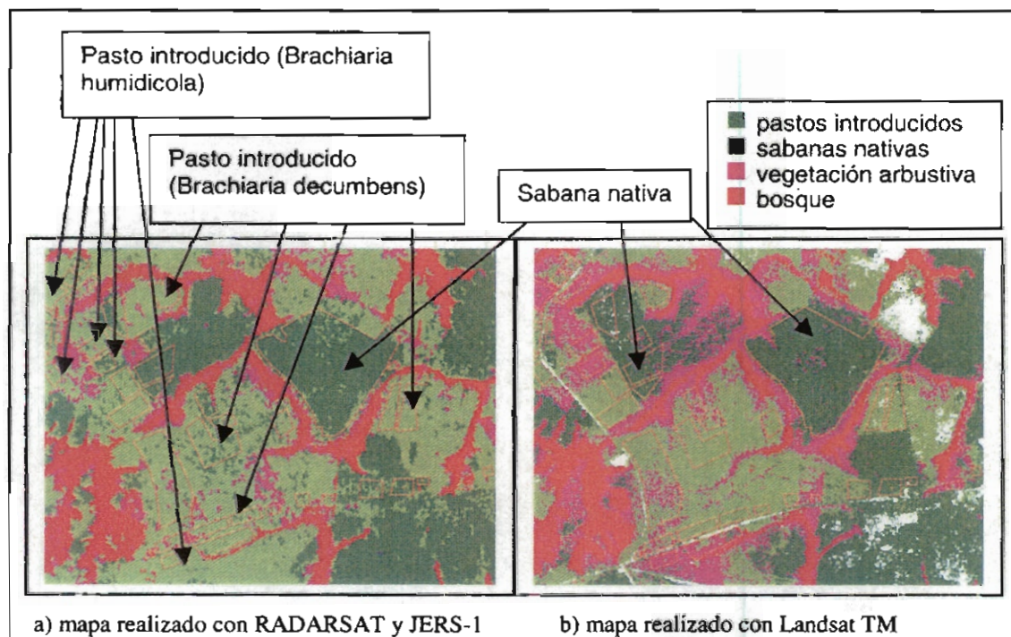
Figura 2: Acercamiento a los dos mapas de uso de la tierra, en una zona de relieve casi plano, con el perímetro de algunas de las parcelas levantadas en 1997 y 1998 indicado en anaranjado.
