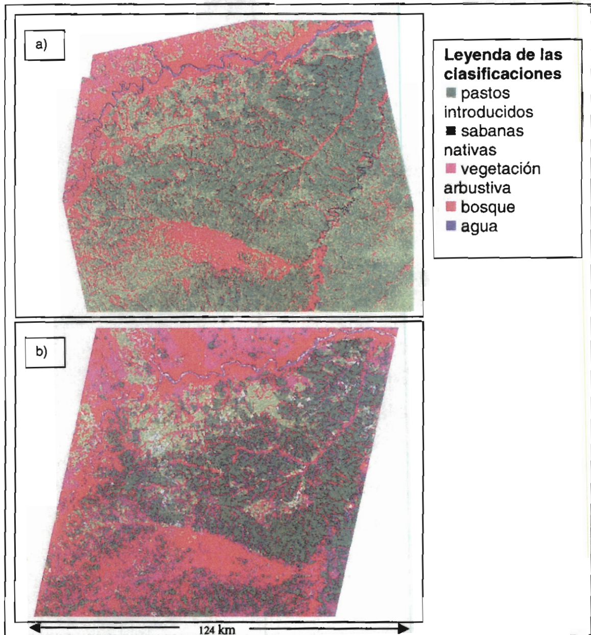
Figura 1: mapas de uso de la tierra realizados con a) imágenes de RADARSAT y JERS-1, según los umbrales de la tabla 2, y b) una clasificación de una imagen Landsat TM de enero de 1988.
