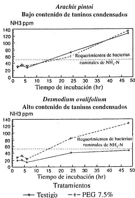
Figura 4.1 Niveles de amonía (NH 3 -N) in vitro en diferentes tiempos de incubación de especies de leguminosas que varían en su contenido de taninos condensados, con o sin PEG.
