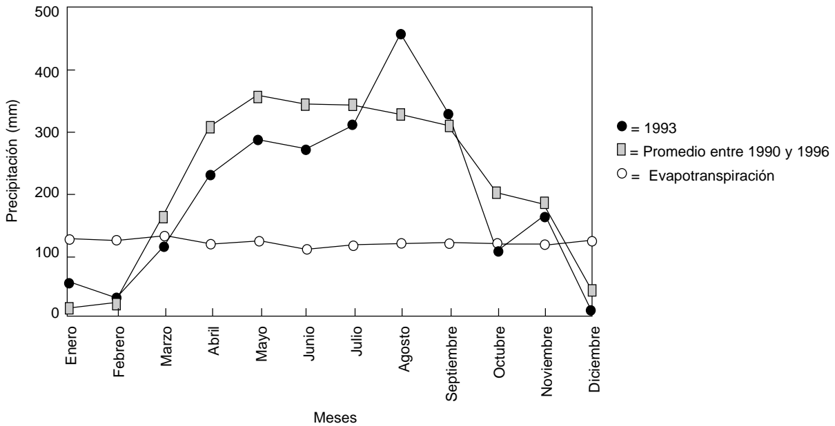
Figura 1. Distribución de la precipitación durante 1993 y entre 1990 y 1996, promedio de evapotranspiración potencial (1973-1994). Hacienda Matazul, Altillanura colombiana.
