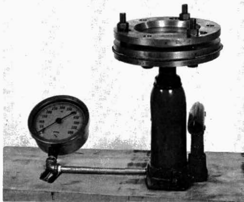
Figura 32. Prensa hidráulica Cambell-Brewster adaptada.
