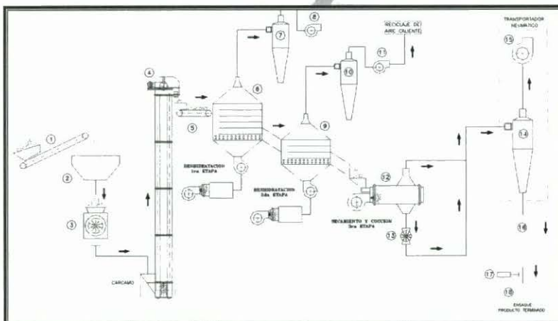
Diagrama típico de flujo. Proyecto: deshidratación industrial para yuca – proceso continuo. Capacidad: 3 ton yuca fresca.
