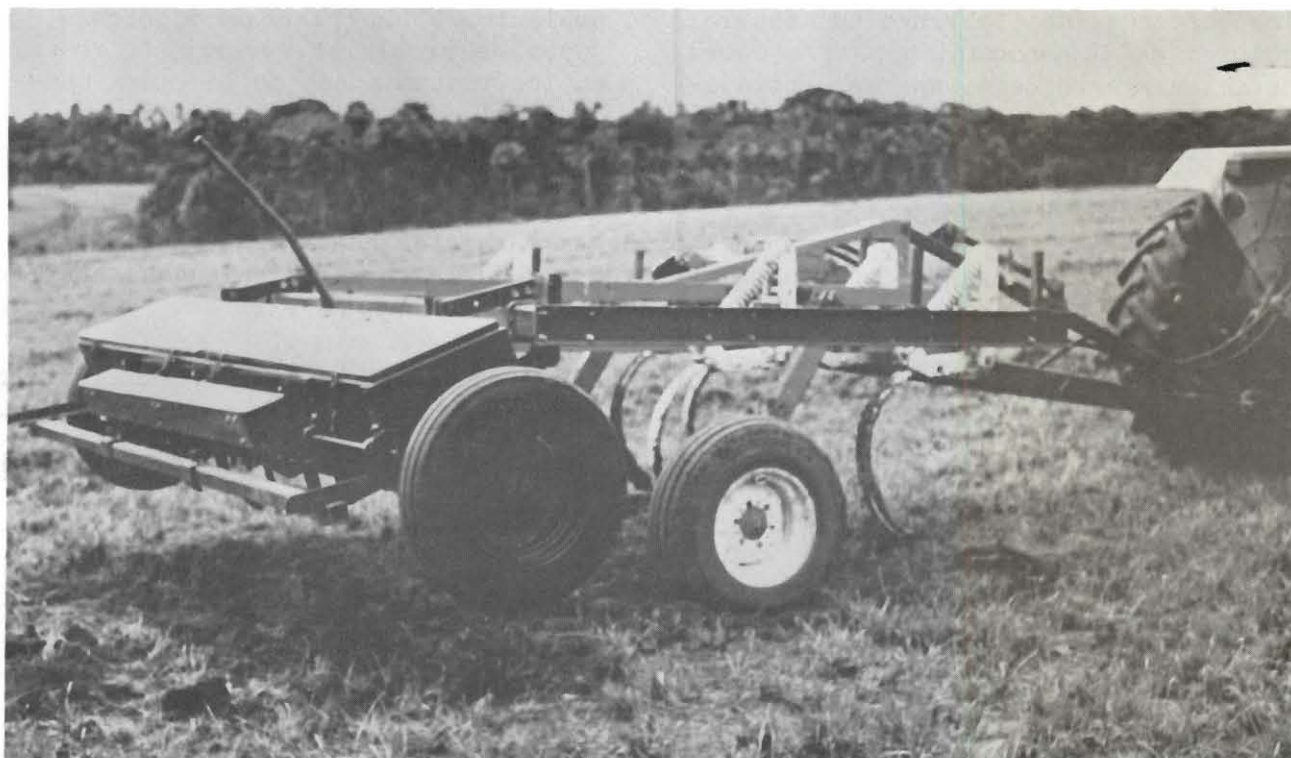
Figura 7. Una sembradora "combinada" que consiste en un arado de cinceles, una abonadora de tolva y una sembradora para semillas pequeñas, utilizada en la siembra de franjas a escala comercial en Carimagua, 1984.
