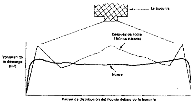
Figura 6-1. Comparación del patrón de aspersión de una boquilla nueva con una usada.
