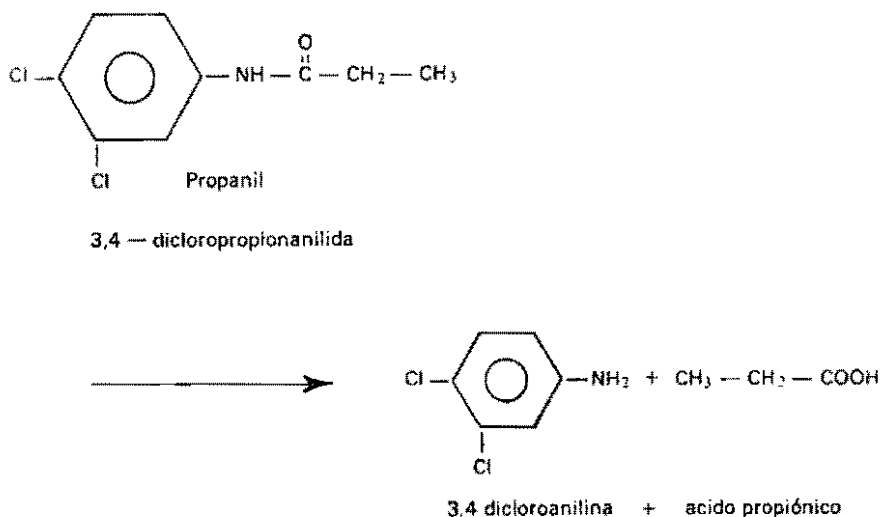
Figura 7-7. Detoxificación del propanil en arroz.
