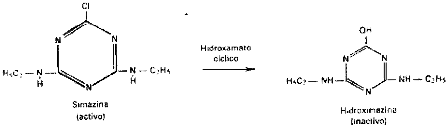
Figura 7-8. Detoxificación de la simazina en maíz
