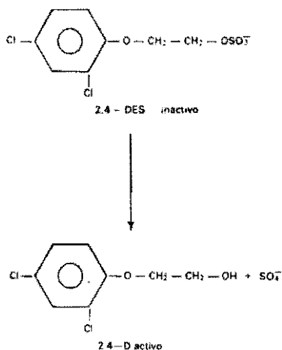
Figura 7-6. Activación del 2,4-DES a 2,4-D en el suelo.
