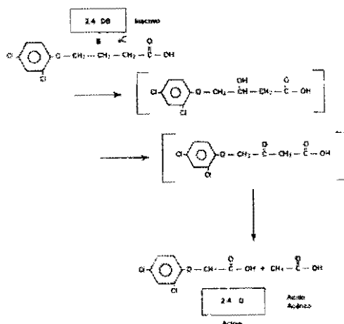
Figura 7-5. Transformación del 2,4-DB a 2,4-D por el proceso de Oxidación beta.
